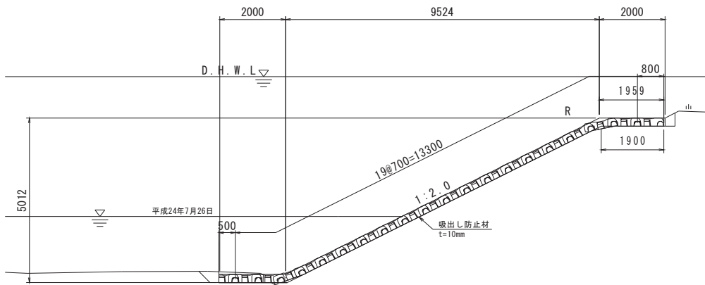
標準断面図
