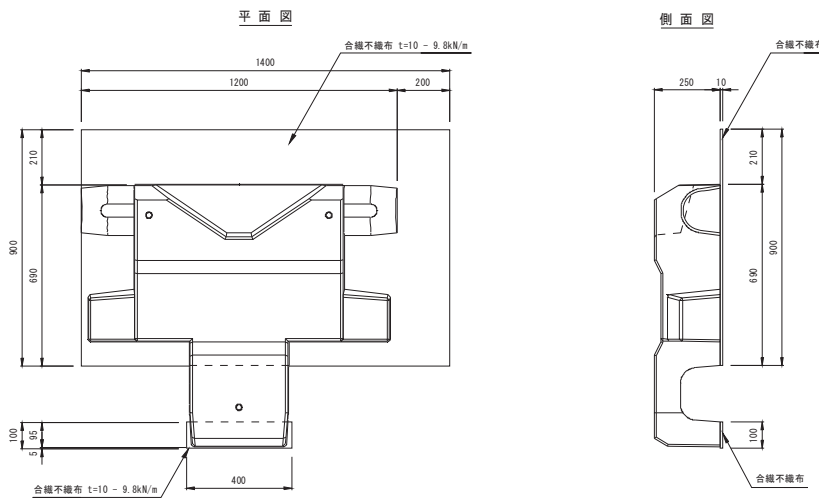
cv 絆 250T B 水中施工用 製品図
